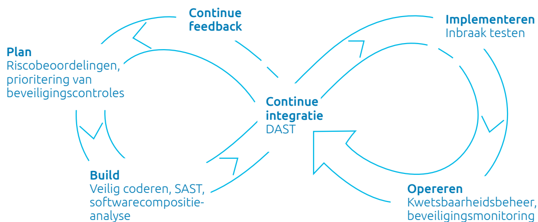
Afbeelding 1: SecDevOps-levenscyclus
